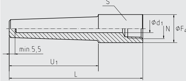
Пример сварного исполнения
