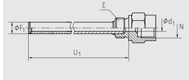
Пример вкручиваемого исполнения
