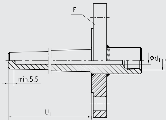
Пример исполнения с фланцем
