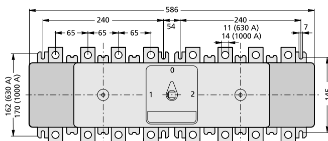
Перекидные выключатели Dumeco, типы DMV 630N и DMV 1000N.
