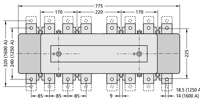
Перекидные выключатели Dumeco, типы DMV 1250N и DMV 1600N.
