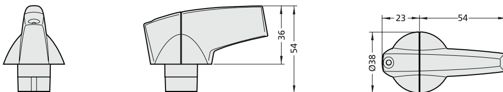
Типы К2А и К2SA.
