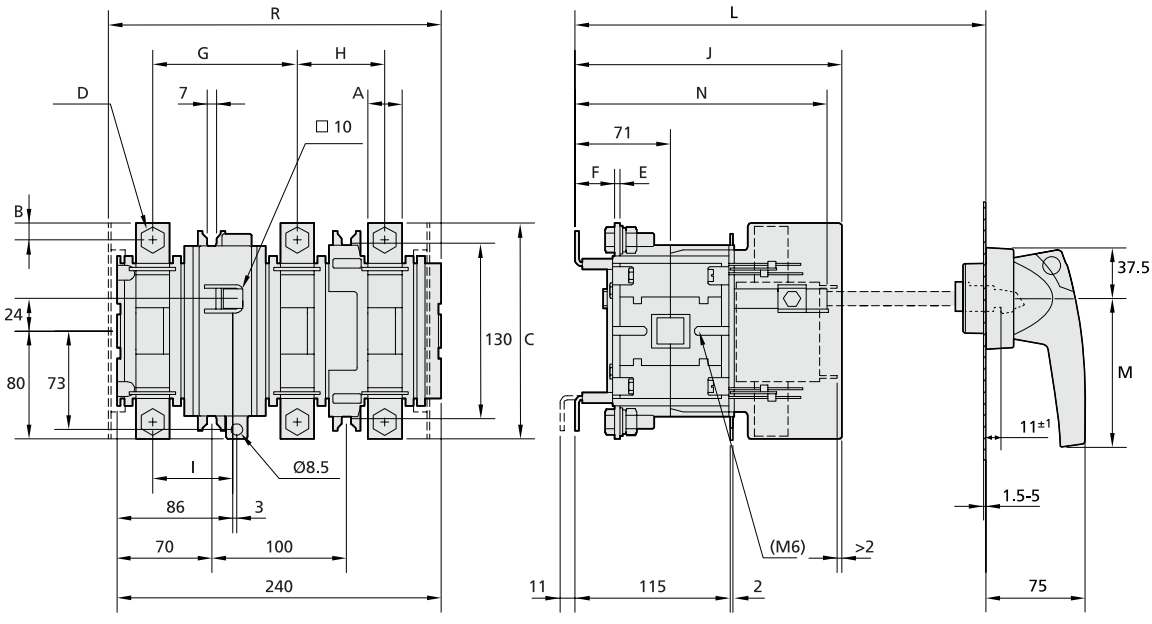
Типы QSA 160N – QSA 400N (DIN).
