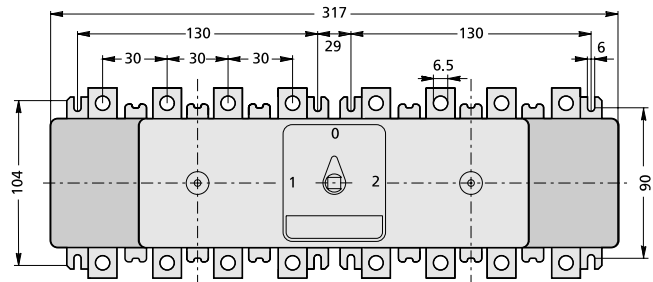
Перекидные выключатели Dumeco, тип DMV 160N.
