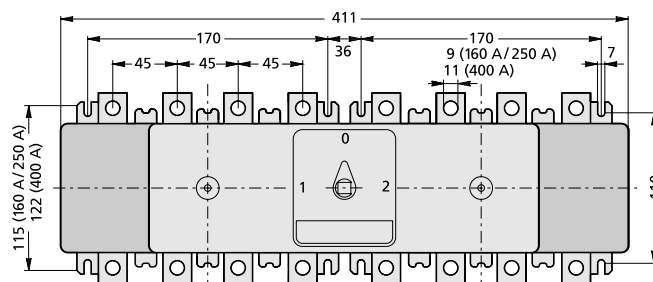
Перекидные выключатели Dumeco, типы DMVS 160N, DMV 250N и DMV 400N.
