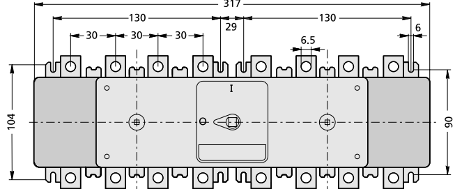
Многополюсные выключатели Dumeco, тип DMV 160N.
